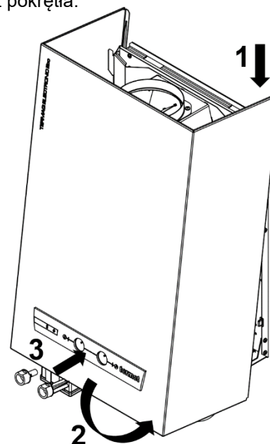
Rys. 3.7.2. Zakładanie osłony przedniej
