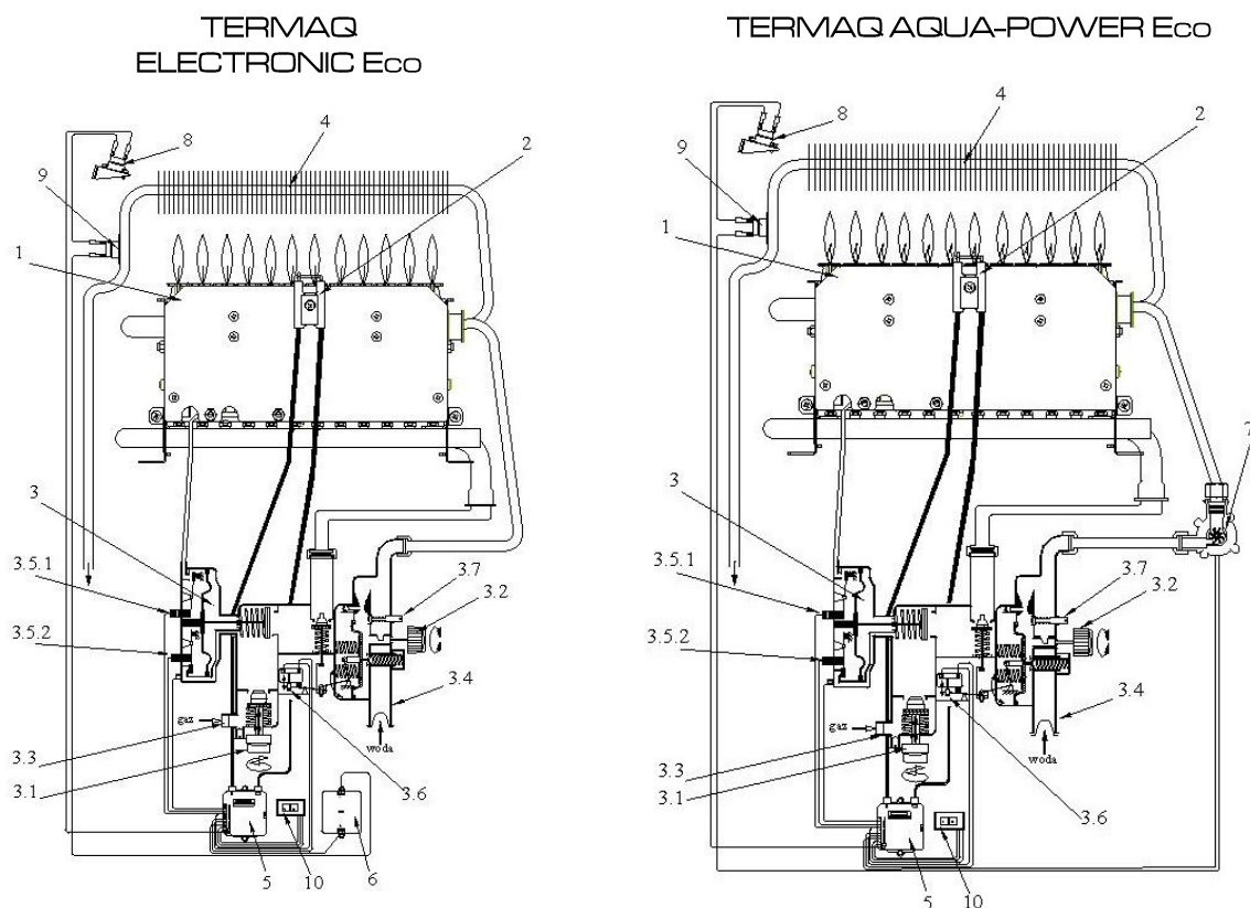
Rys. 2.2.1.2 Schemat ideowy ogrzewacza
