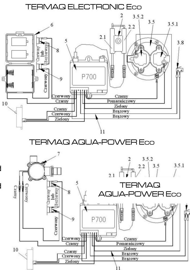
Rys 2.2.1.3 Schemat elektryczny ogrzewacza
