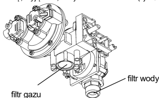
Rys.6.4.1 Armatura wodno-gazowa
